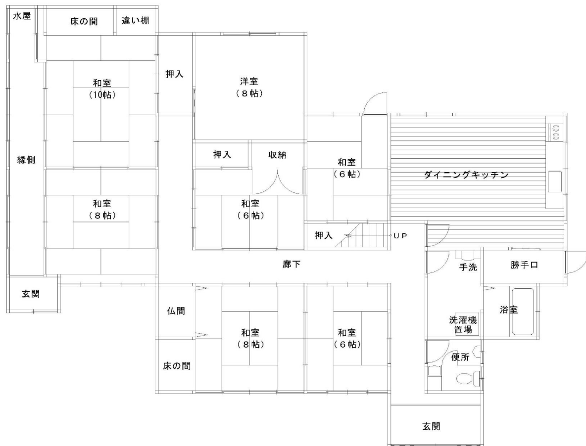
1 階平面図
